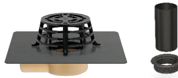
SitaCompact abgewinkelt DN 70 mit SitaCompact Anstauring
